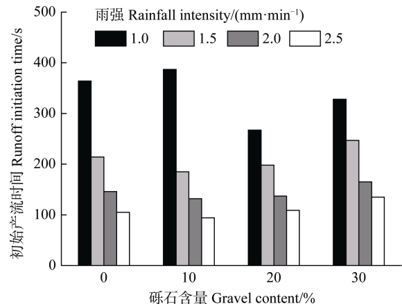
图 1 初始产流时间随砾石含量和雨强的变化
