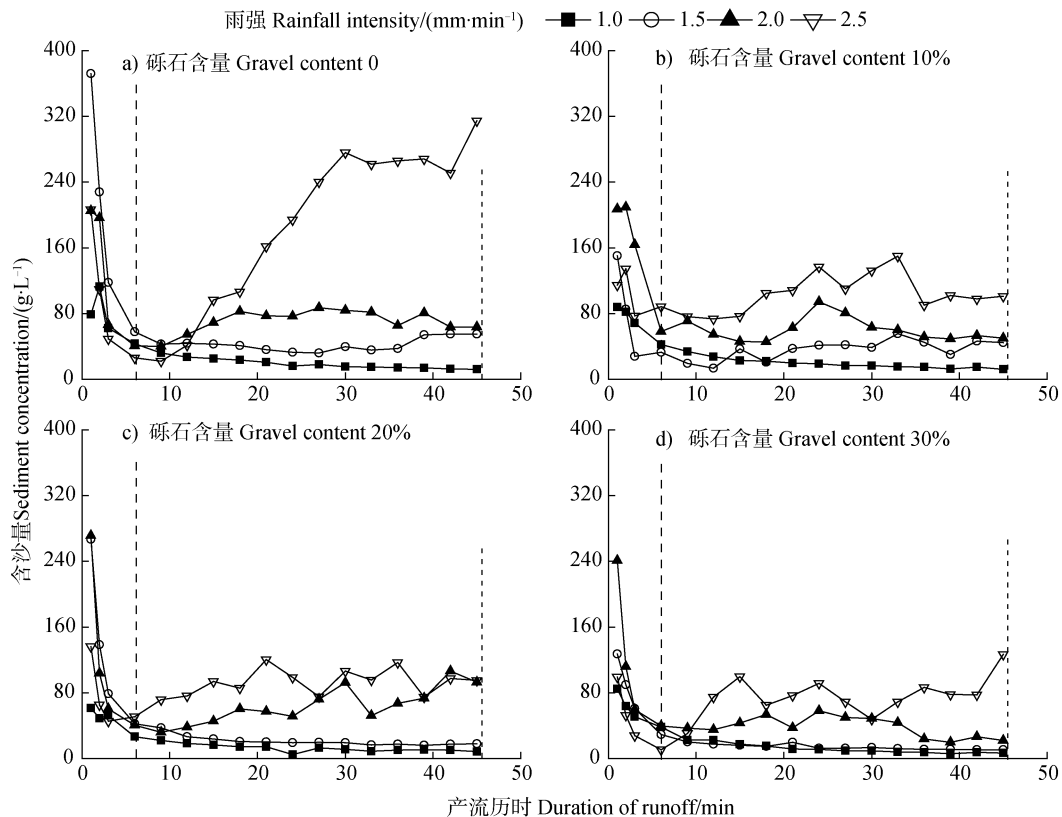
图 4 不同砾石含量和雨强条件下含沙量随产流历时的变化
