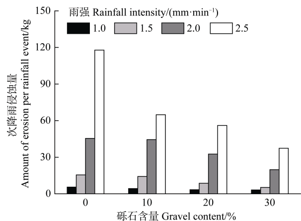
图 5 次降雨侵蚀量随砾石含量、雨强的变化
