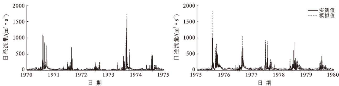
图 1 泾河流域景村水文站 1970—1979 年日径流模拟结果
