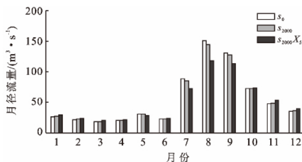
图 2 梯田对泾河流域月均径流的影响
