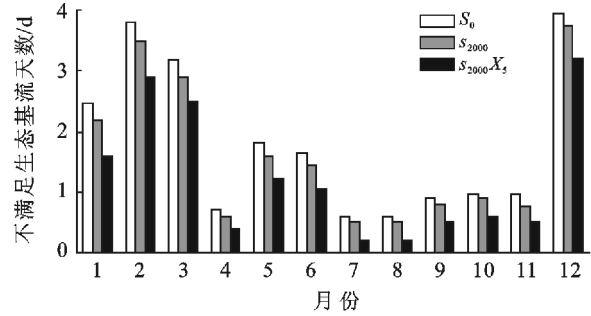
图 5 梯田措施对泾河流域月生态基流保障的影响
