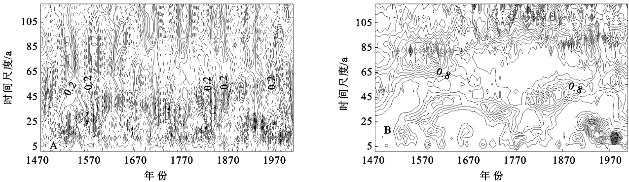
图 3 兰州地区小波分析的系数分布
