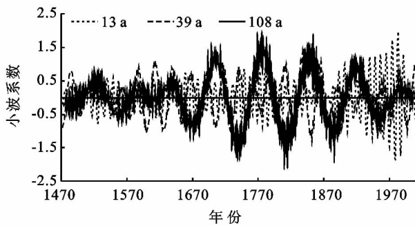
图 5 兰州地区 13 a、39 a 及 108 a 周期的小波系数时间序列对比
