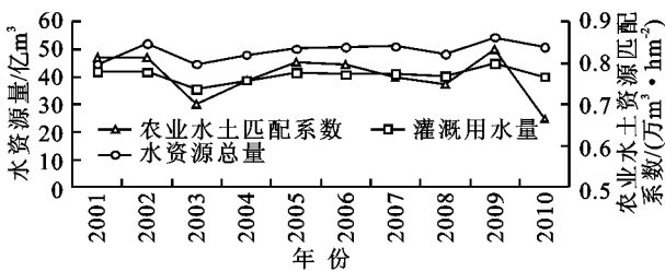
图 1 河套灌区农业水土资源匹配系数与水资源总量变化趋势对比
