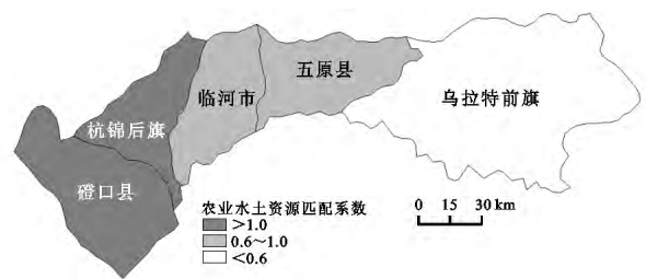
图 2 2010 年河套灌区农业水土资源匹配空间格局
