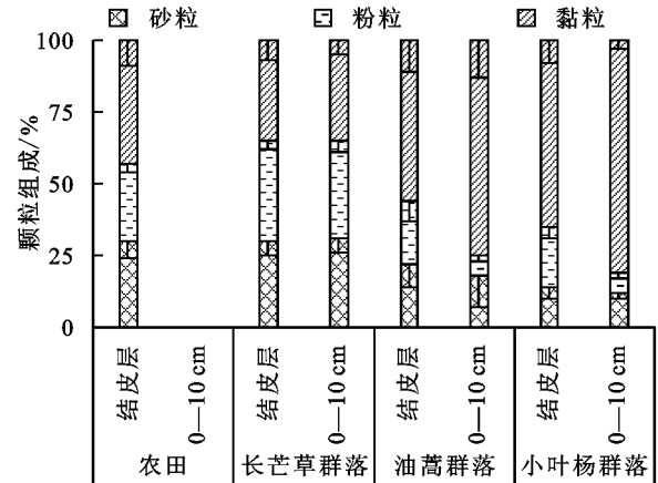
图 1 不同植被群落生境下生物结皮的叶绿素含量和土壤颗粒组成
