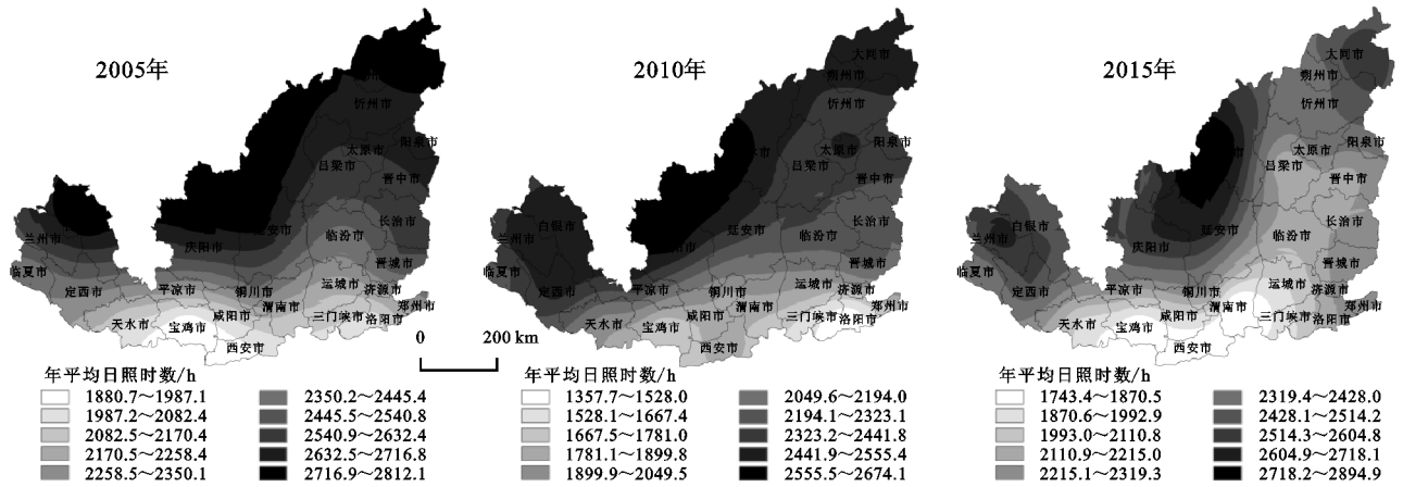
图 7 黄土高原苹果主产区 2005 年、2010 年和 2015 年年平均日照时数区域变化差异
