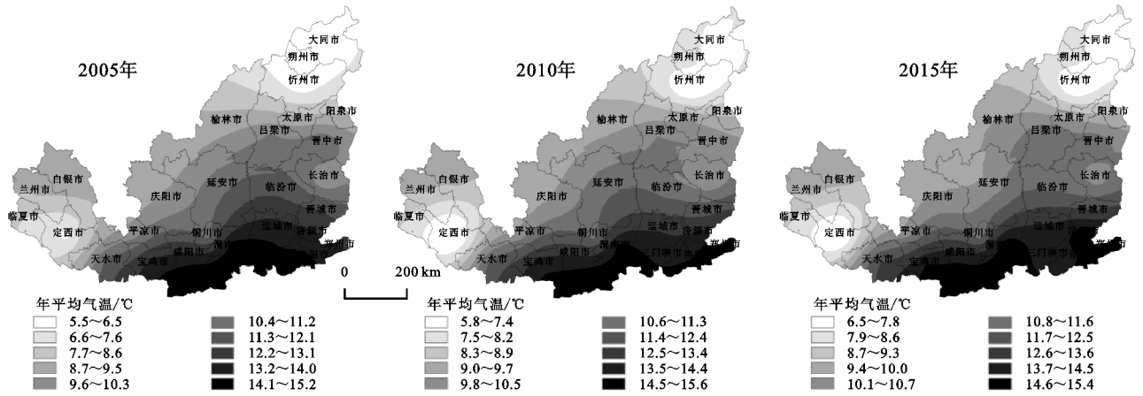
图 6 黄土高原苹果主产区 2005 年、2010 年和 2015 年年平均气温区域变化差异
