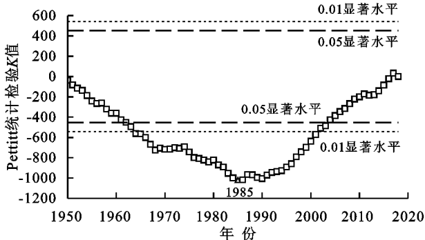
图 3 潼关水文站年径流量变化趋势 Pettitt 检验
