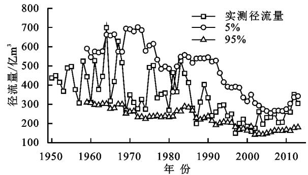
图 5 潼关水文站不同频率径流量年际变化过程
