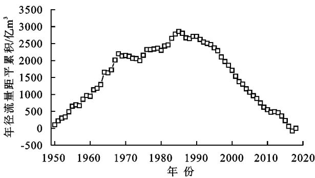
图 4 潼关水文站年径流量距平累积曲线
