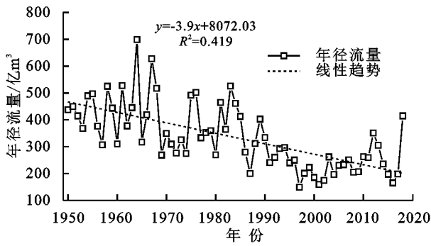
图 2 潼关水文站年径流量变化及其趋势
