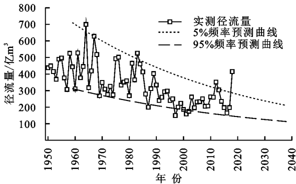
图 6 潼关水文站实测年径流量及不同频率预测区间
