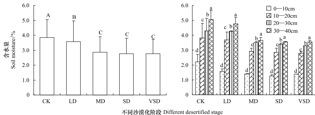
图2 不同沙漠化阶段草地土壤含水量及其垂直分布特征
