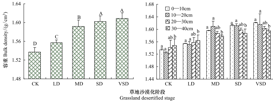
图 3 不同沙漠化阶段草地土壤容重变化及其垂直分布特征
