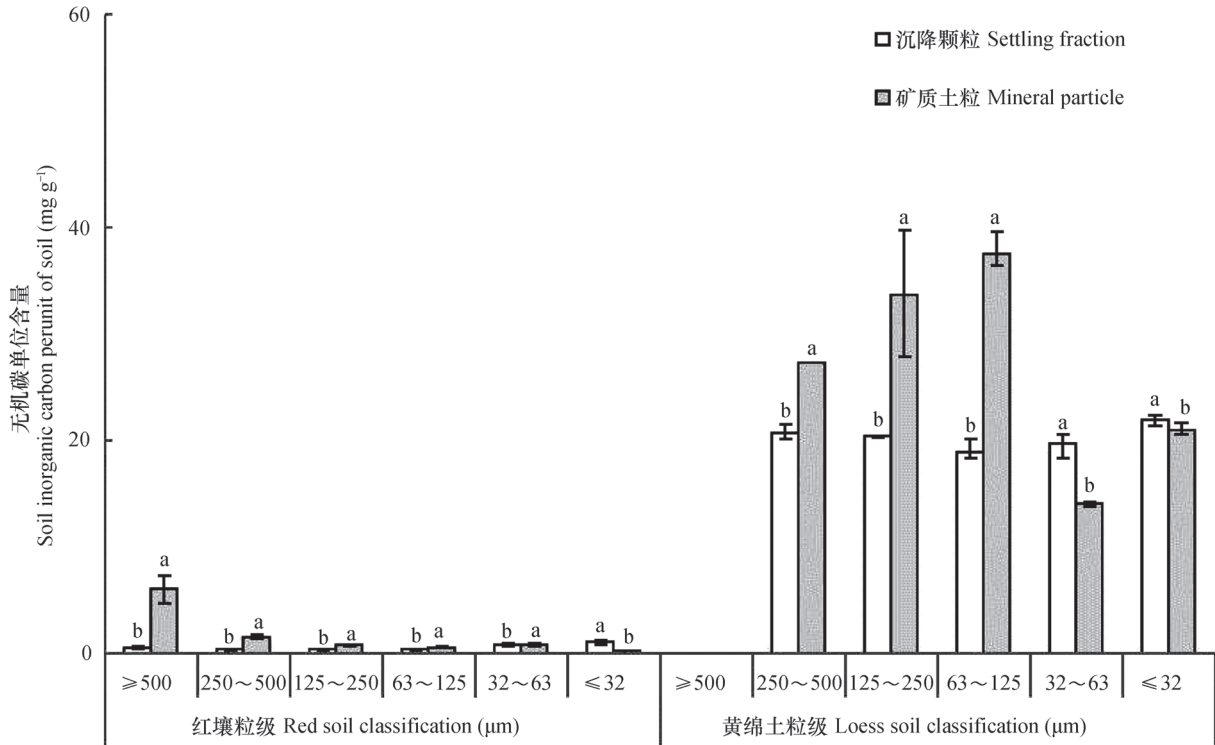
图5 无机碳单位含量在红壤和黄绵土不同沉降速度和矿质粒度中的分布
