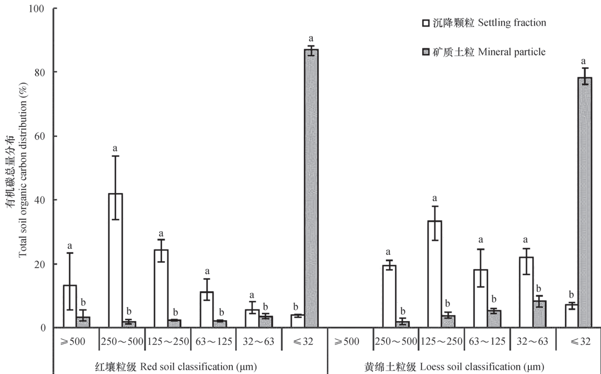
图4 有机碳总量在红壤和黄绵土不同沉降速度和矿质粒径中的分布
