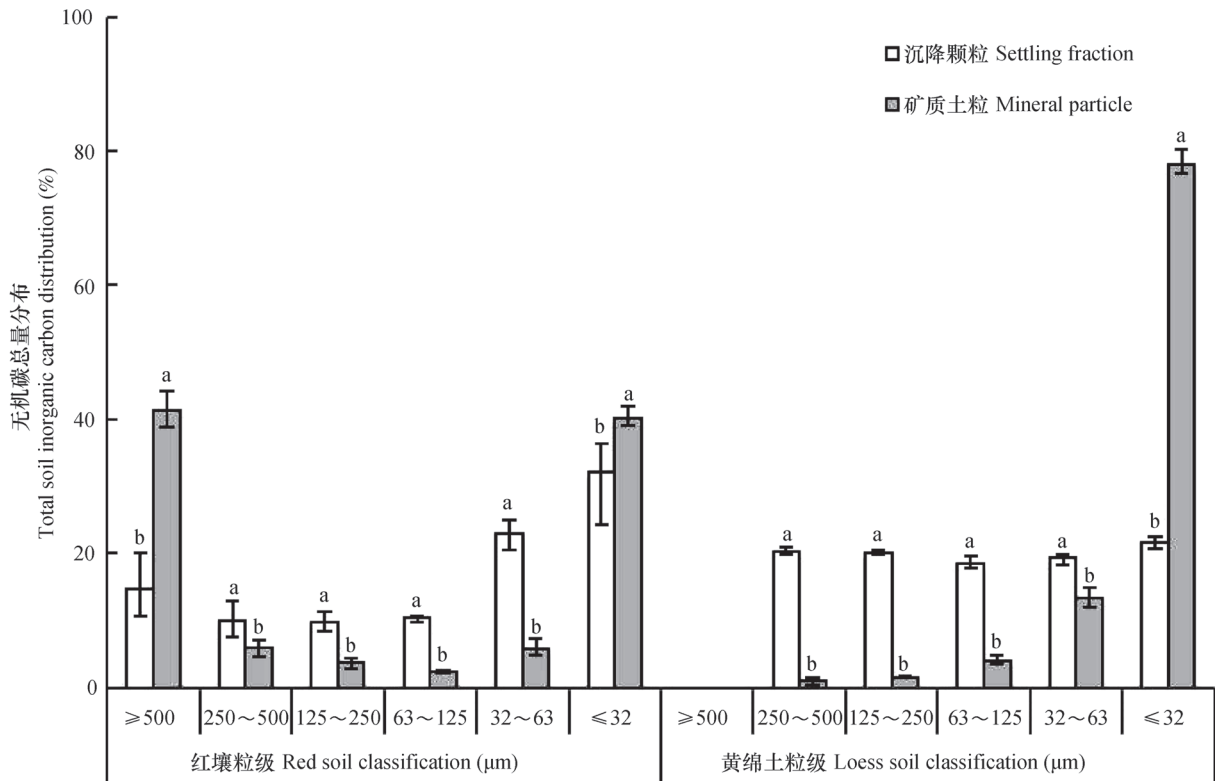
图6 无机碳总量在红壤和黄绵土不同沉降速度和矿质粒度中的分布
