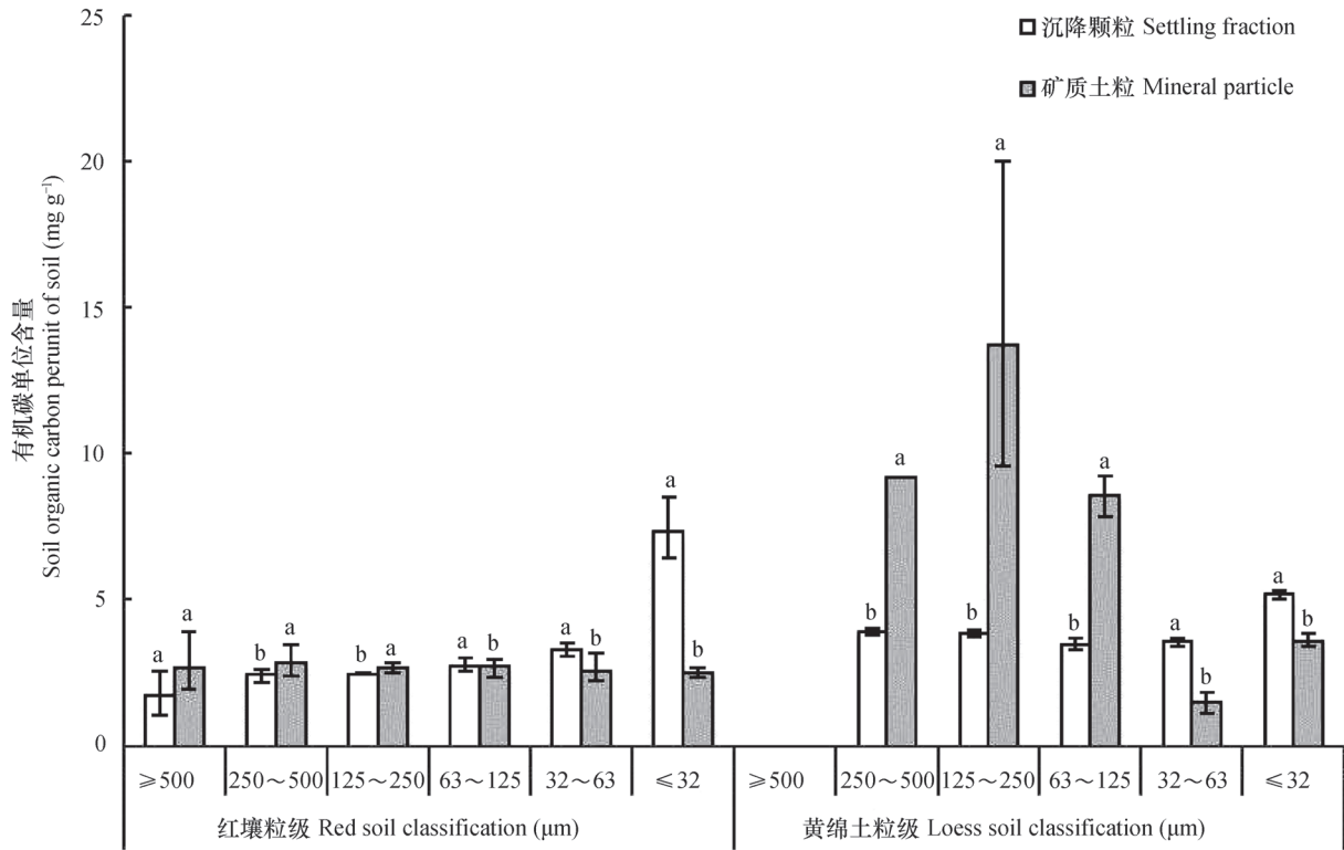
图3 有机碳单位含量在红壤和黄绵土不同沉降速度和矿质粒径中的分布
