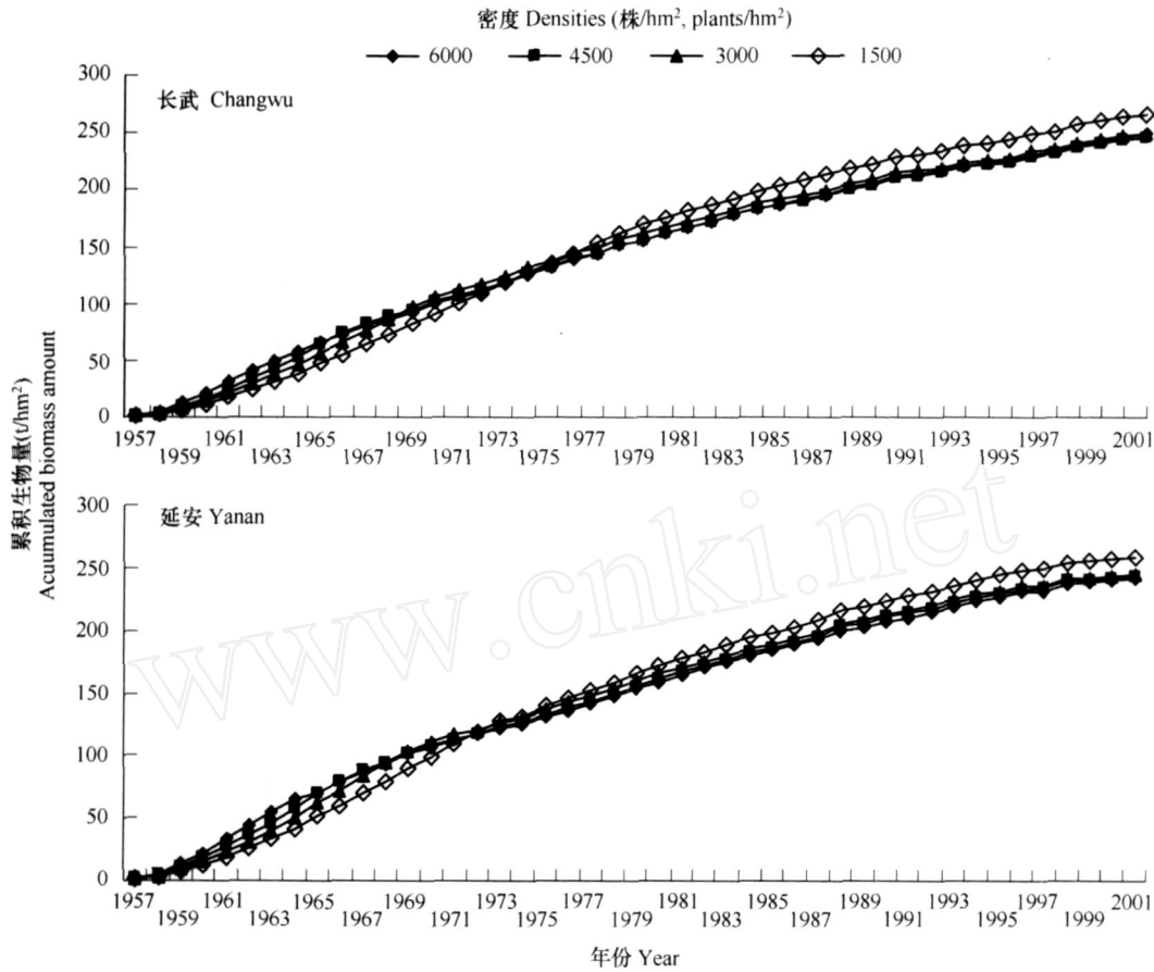
图3 长武和延安不同密度刺槐林地累积生物量模拟值比较
