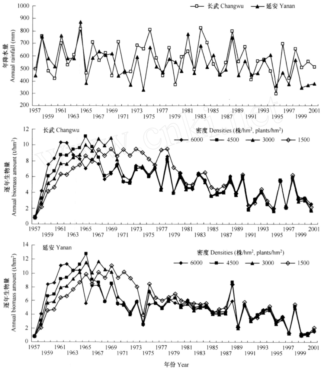
图 2 长武和延安年降水量和不同密度刺槐林地逐年生物量模拟值比较
