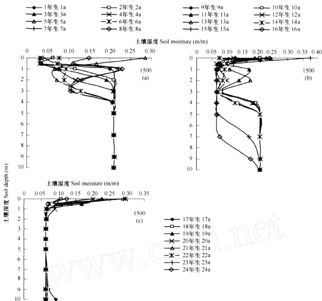
图 9 延安不同密度刺槐林地 0~10m 土层土壤湿度剖面分布年度变化比较
