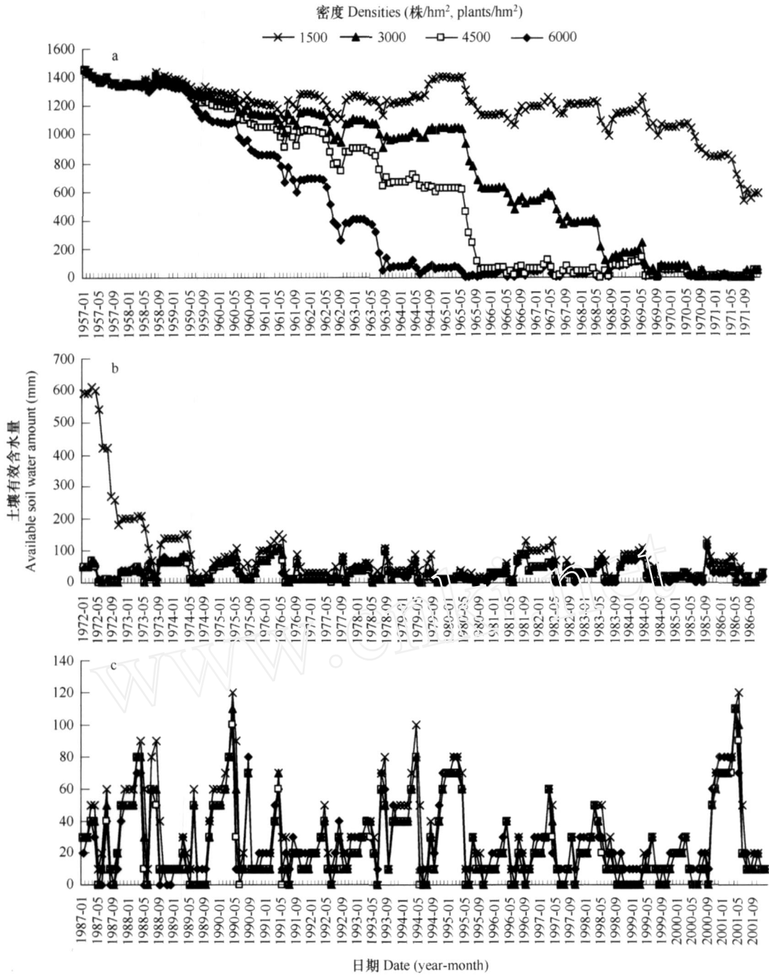
图 7 延安不同密度刺槐林地 0~10m 土层逐月土壤有效含水量模拟值比较
