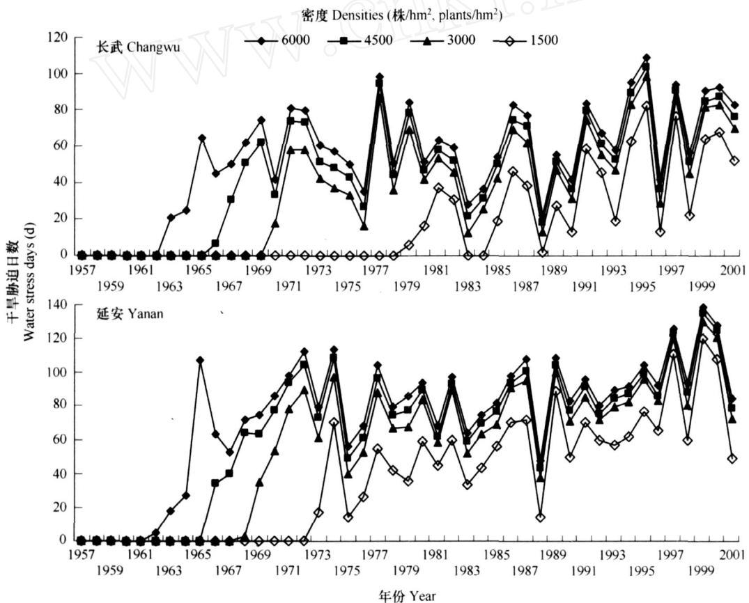
图 5 长武和延安不同密度刺槐林地干旱胁迫日数模拟值比较
