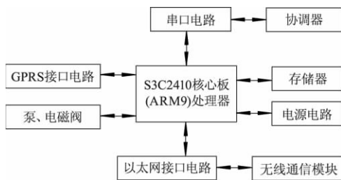
图 3 基站结构图
