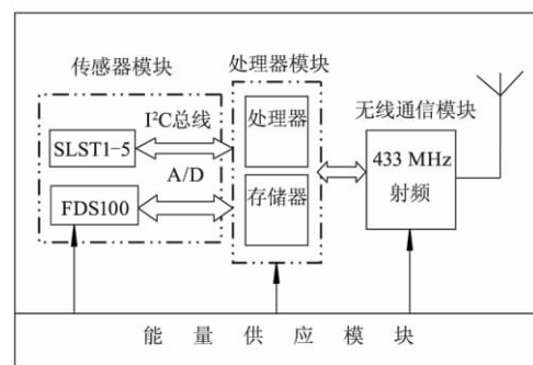
图 2 无线传感器网络节点的体系结构
