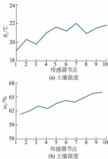
图 6 采集的土壤温度和湿度
