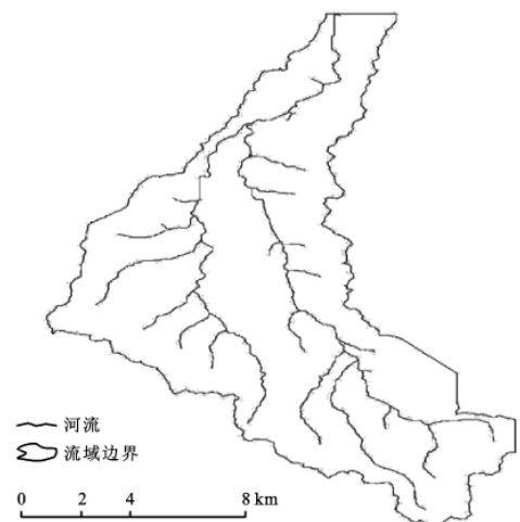
图 4 基于 DEM 提取的河网
