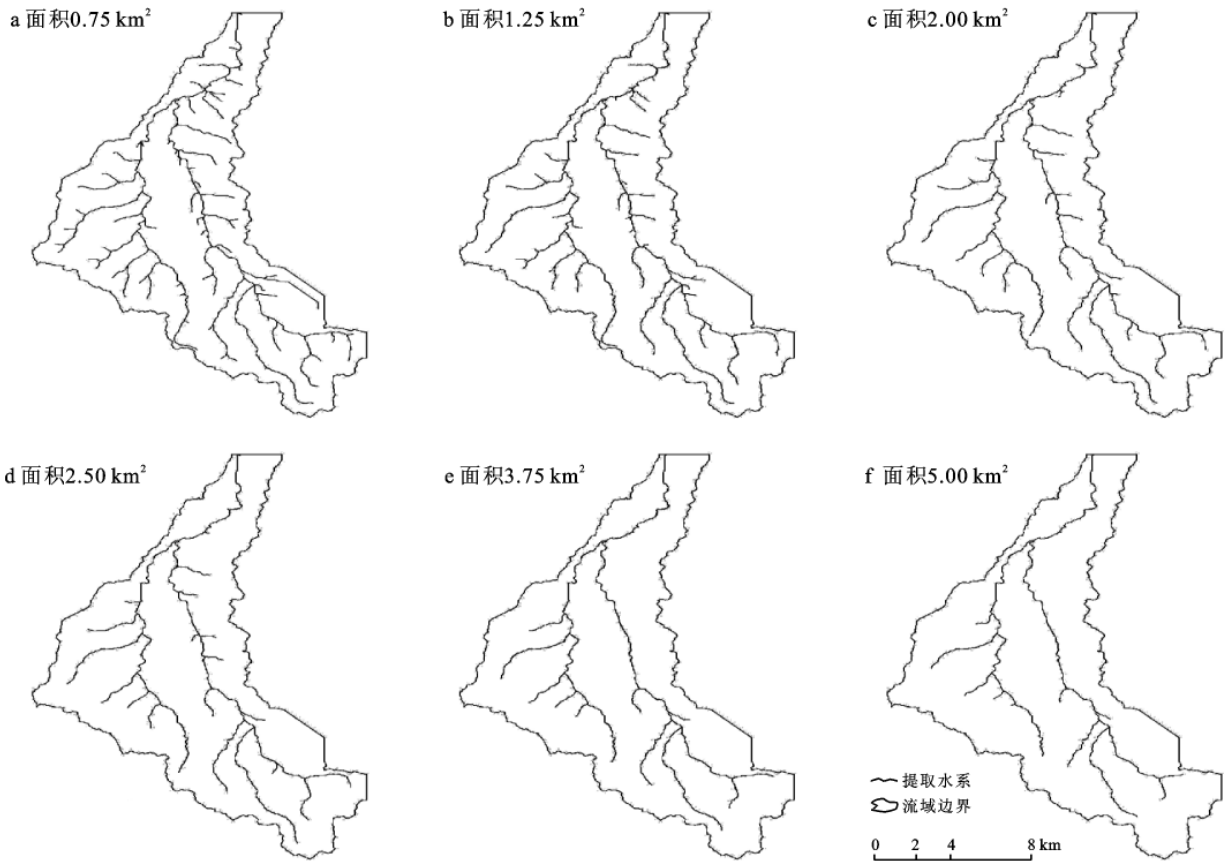
图 1 流域河网随集水面积阈值变化
