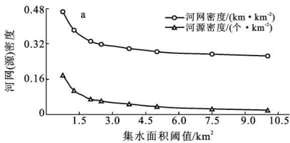
图 2 河网密度、河源密度与集水面积阈值的关系
