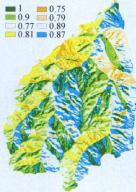
图6 坡向系数
