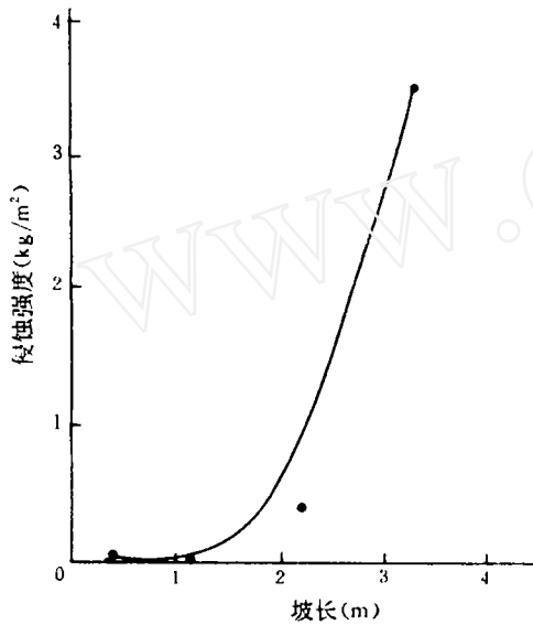
图2 1 # 模型侵蚀强度分布趋势 ( I = 1.14\text{mm/min} )
