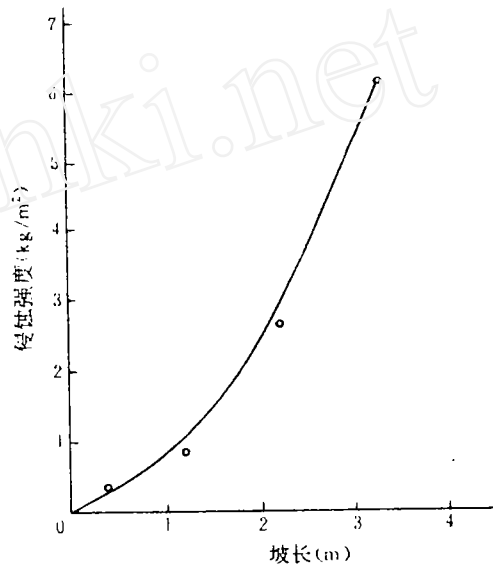
图3 2 # 模型侵蚀强度分布趋势 ( I = 1.14\text{mm/min} )
