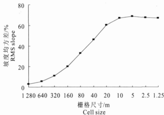
图1 坡度均方差与栅格尺寸关系曲线
