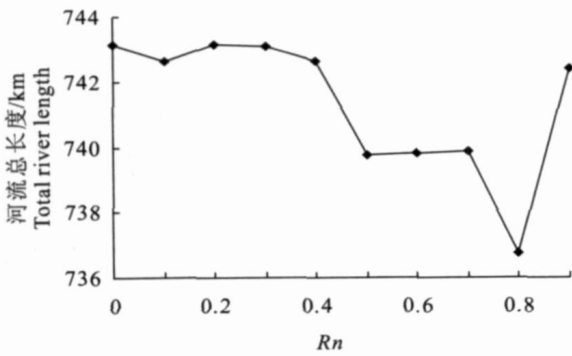
图6 R_n 对提取河流总长度的影响
