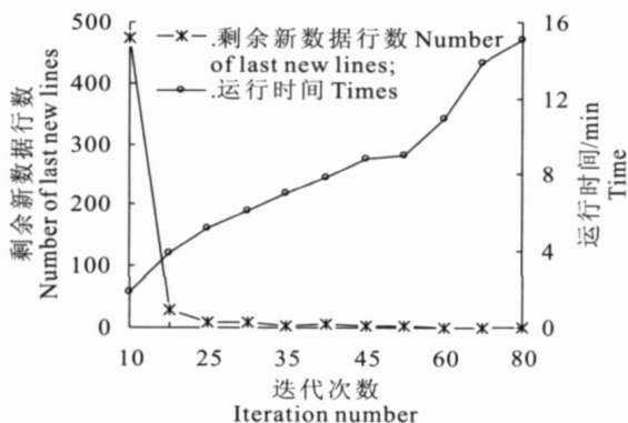
图2 迭代次数对剩余新数据行数和运行时间的影响
