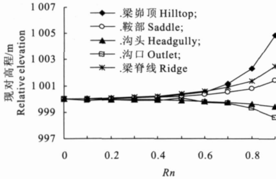
图4 R_n 对地貌特征的影响
