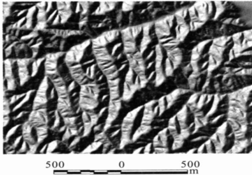
图9 ANUDEM建立的DEM光照模拟图 Fig. 9 Hillshade of the constructed DEM
