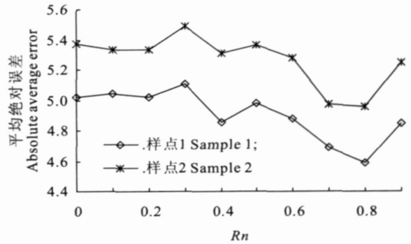
图7 R_n 对高程平均绝对误差的影响
