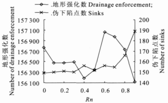
图5 R_n 对地形强化数和伪下陷点数的影响
