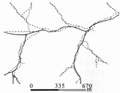
图11 基于不同DEM提取的水系网络图
