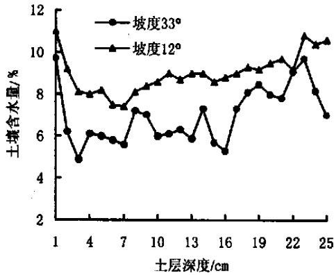
图1 不同坡度刺槐林地土壤水分状况
