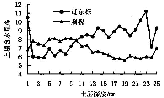
图2 天然林与刺槐人工林地土壤水分
