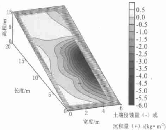
图 3 土壤侵蚀强度空间分布
