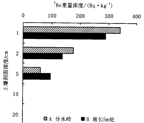
图 2 7 Be 在土壤剖面中的分布
