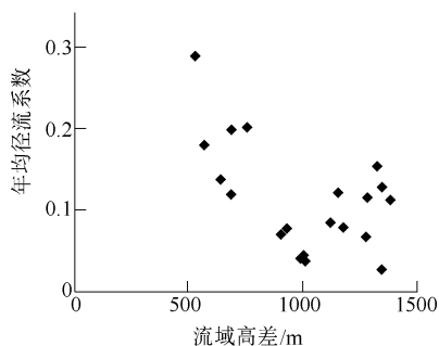
图7 年均径流系数与流域高差关系
