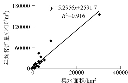
图 1 年均径流量与集水面积关系
