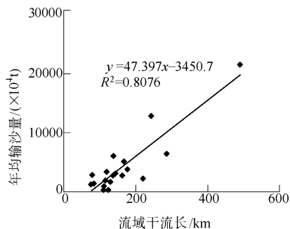
图 12 年均输沙量与流域干流长关系
