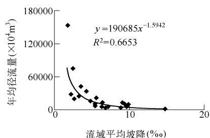
图 2 年均径流量与流域平均坡降关系
