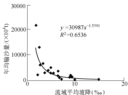
图 10 年均输沙量与流域平均坡降关系
