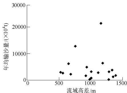
图 11 年均输沙量与流域高差关系
