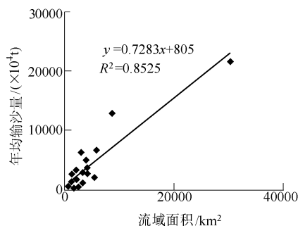
图 9 年均输沙量与流域面积关系
