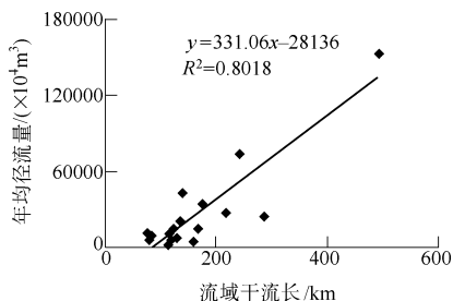
图4 年均径流量与流域干流长关系
