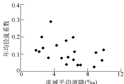
图6 年均径流系数与流域平均坡降关系
