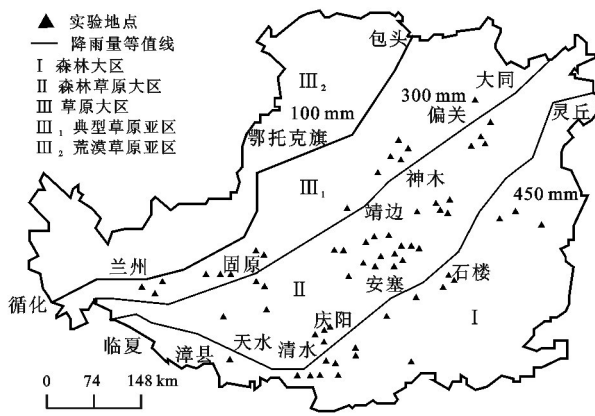
图 1 黄土高原分区与研究样点分布
