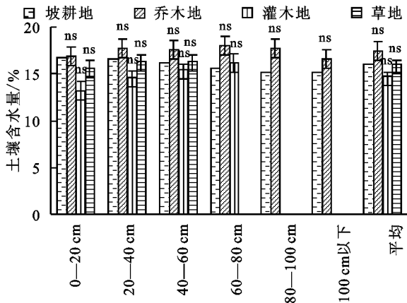
图 4 森林区坡耕地退耕为乔、灌、草土壤剖面水分变化
