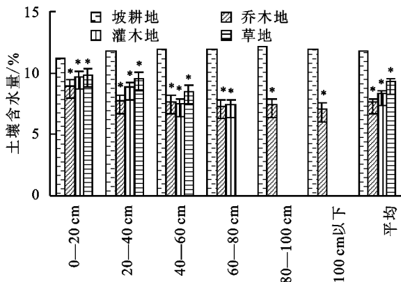
图 3 森林草原区坡耕地退耕为乔、灌、草土壤剖面水分变化
