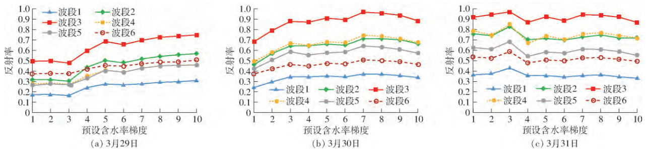
图5 土样光谱反射率随含水率变化关系曲线
