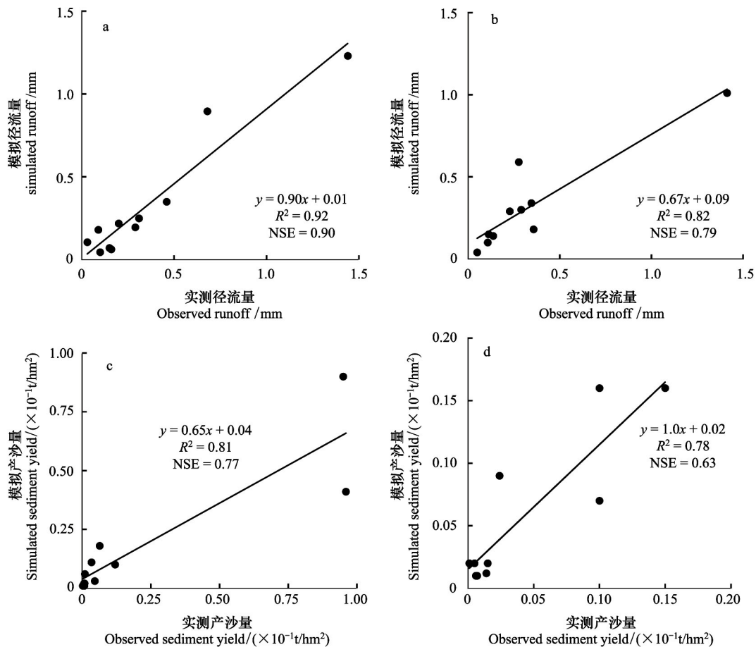
图 1 土壤参数率定结果验证
