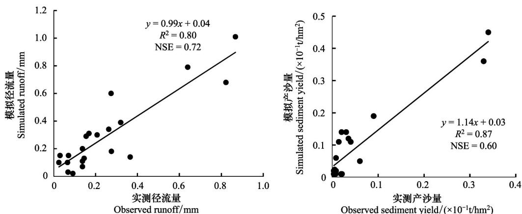
图 2 验证水平阶有效性
