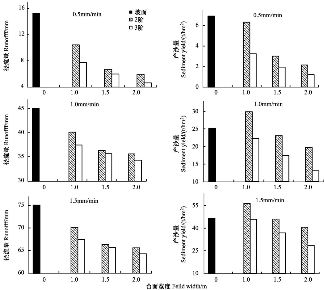
图 4 不同雨强下产流产沙量随不同水平阶规格的变化
