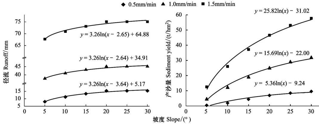
图 3 不同雨强下坡度变化对产流产沙的影响
