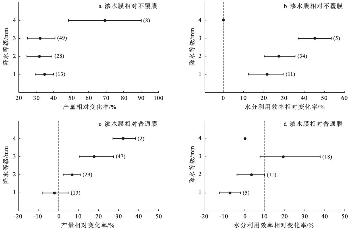
图 5 不同年降水量下渗水地膜对不同作物产量和水分利用效率(WUE)的影响
