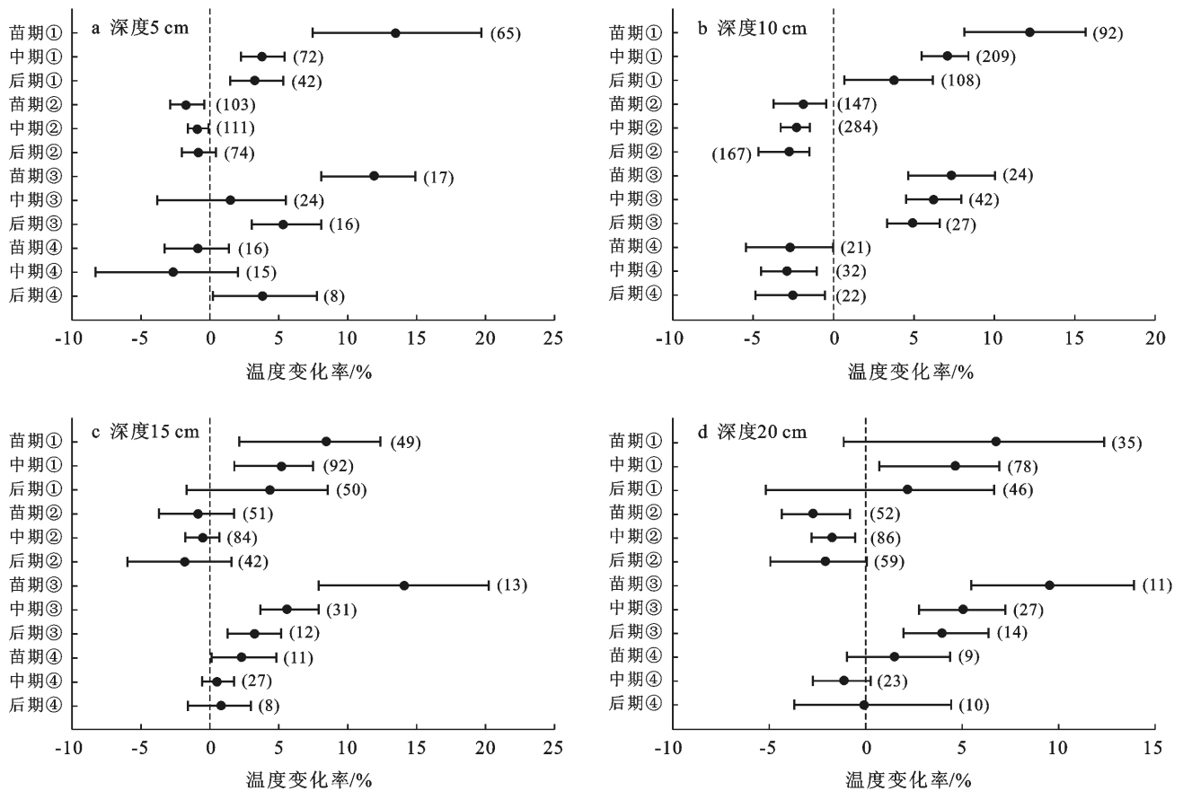
图 6 降解地膜或渗水地膜相对不覆盖或普通地膜覆盖对不同深度土壤温度的影响
