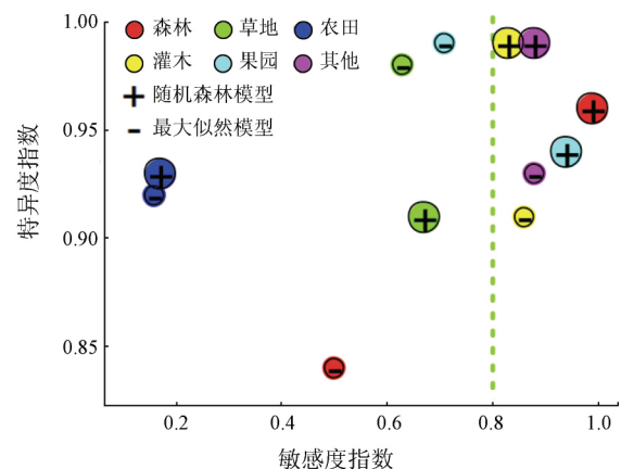
图 2 随机森林和最大似然模型的 6 种土地利用的敏感度和特异度指数
